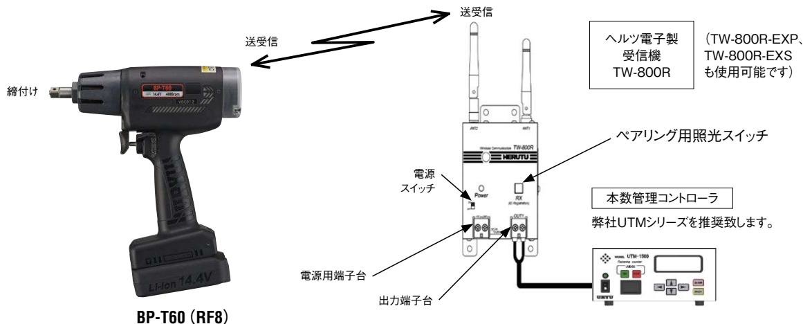
RF8: ポカヨケシステム図
