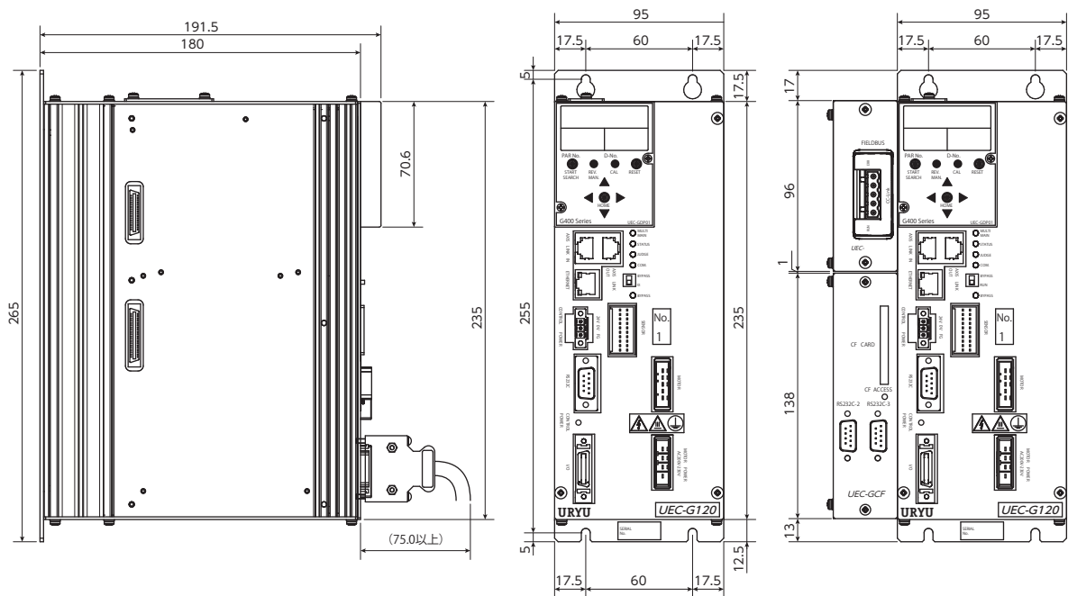
UEC-G120 外観図 (mm)
